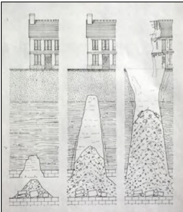
Formation et évolution d'un fontis © Marc Viré
